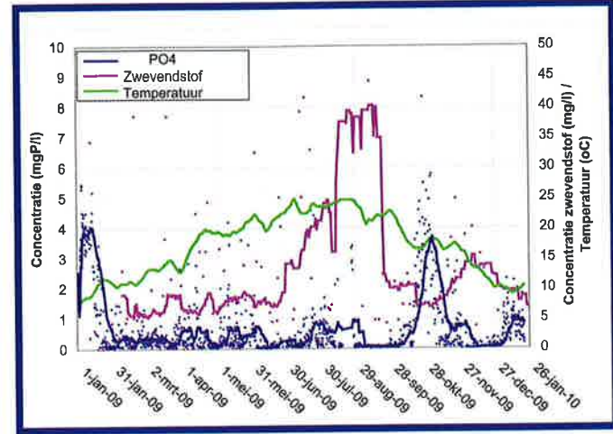
Afb. 4: Epe reactor 2: effluentconcentraties fosfaat, zwevendstof en temperatuur.v
